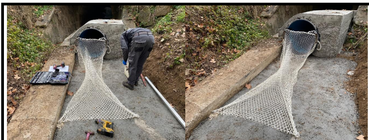
Instalación de 1 cesta Tecno-Grabber® en un colector de ø800mm. El Pont de Vilomara i Rocafort (Barcelona). Cortesía de Tecnoconverting.
