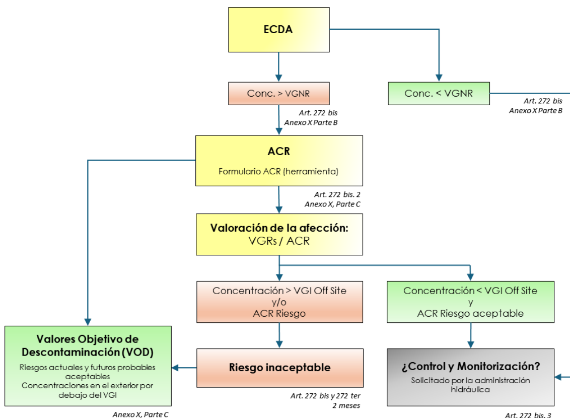
Figura 13. Diagrama de proceso: ACR, valoración de la afección y actuaciones.
