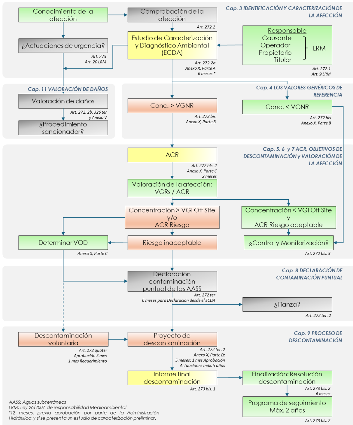
Figura 2. Esquema General del RDPH. Contaminación puntual de las AA.SS.
