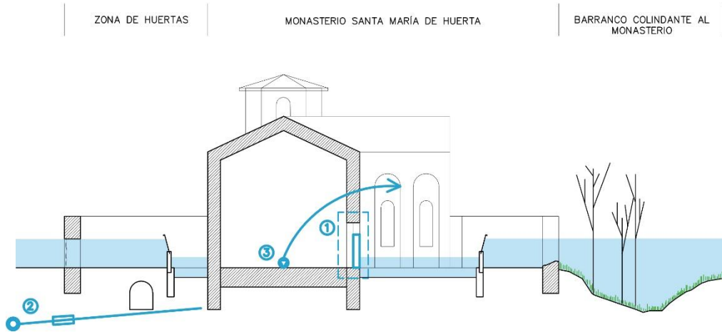
Fig. 52: Medidas complementarias: esquema en sección. 1 barreras temporales, 2 sistemas antirretorno, 3 bombas de achique y SAI.
