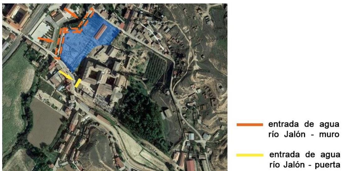
Fig. 26: Entrada de agua en el recinto procedente del río Jalón para el periodo de retorno de 500 años.
