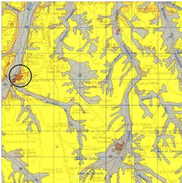
Fig. 14: Mapa Geológico Nacional (Detalle hoja 436). Instituto Geológico y Minero de España.
