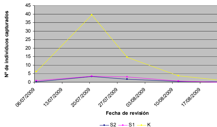
COMPARATIVA FEROMONAS Lymantria dispar QUINTOS DE MORA 2009 - Medias por itinerario zona Z1
