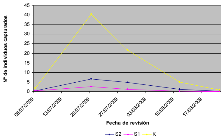
COMPARATIVA FEROMONAS Lymantria dispar QUINTOS DE MORA 2009 - Medias por itinerario zona Z2
