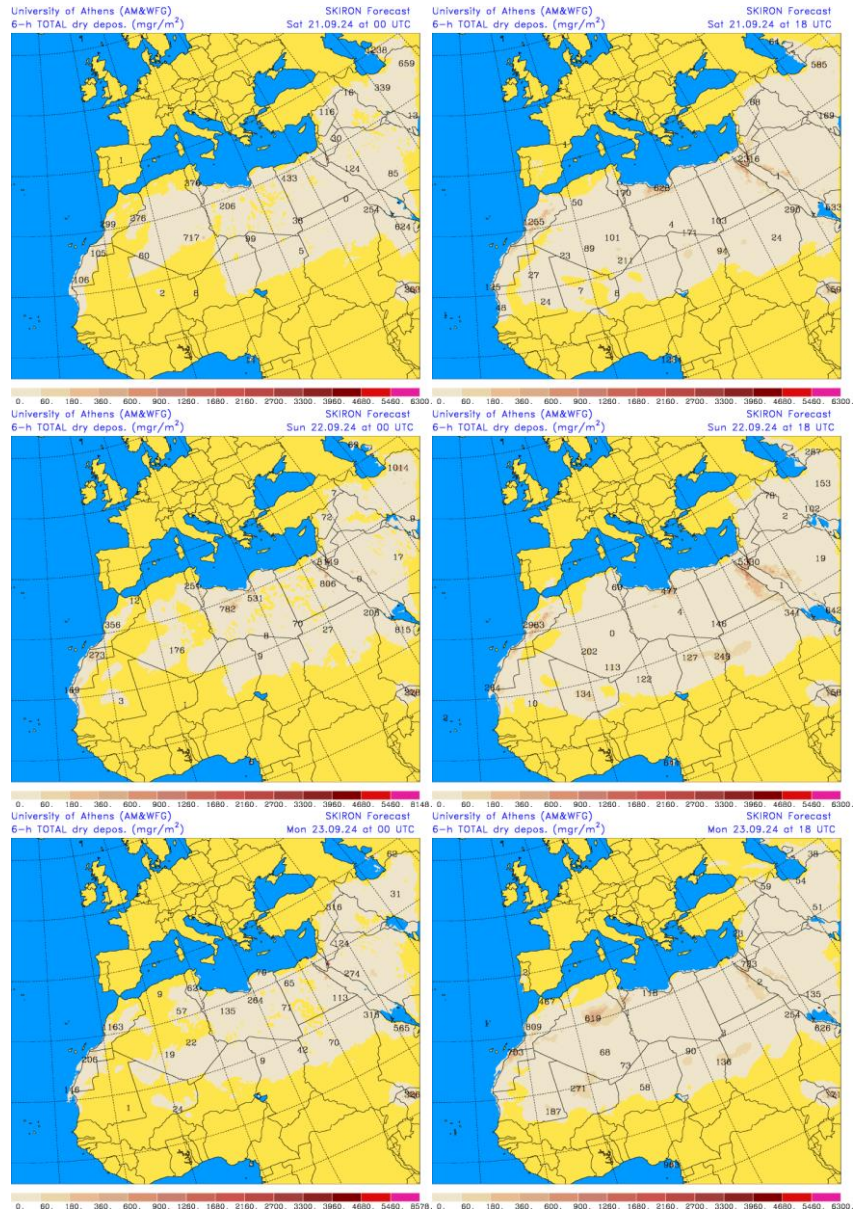
Depósito seco de polvo (mg/m 2 ) predicho por el modelo SKIRON para los días 21, 22 y 23 de septiembre de 2024 a las 00 y 18 UTC © Universidad de Atenas.
