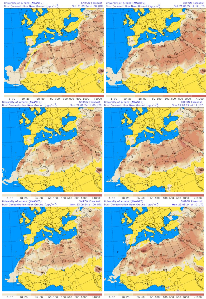
Concentración de polvo ( \mu\text{g}/\text{m}^3 ) predicha por el modelo SKIRON para los días 21, 22 y 23 de septiembre de 2024 a las 00 y 12 UTC © Universidad de Atenas.
