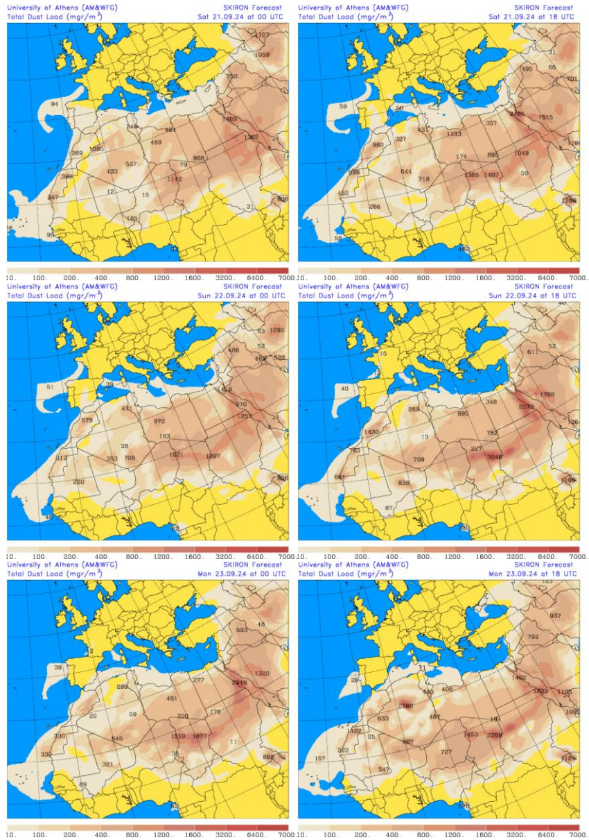
Carga total de polvo (mg/m 2 ) predicha por el modelo SKIRON para los días 21, 22 y 23 de septiembre de 2024 a las 00 y 18 UTC © Universidad de Atenas.
