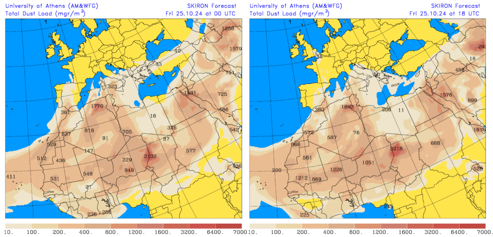
Carga total de polvo (mg/m 2 ) predicha por el modelo SKIRON para el día 25 de octubre de 2024 a las 00 y 18 UTC © Universidad de Atenas.
