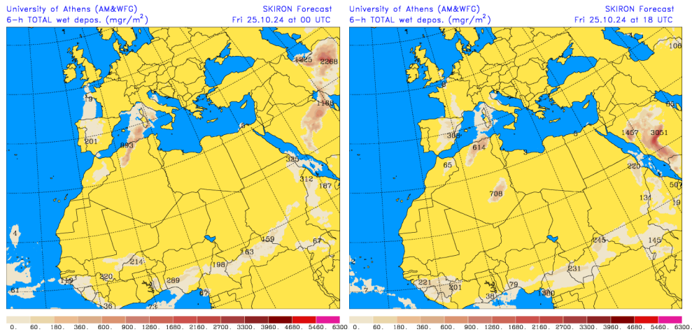
Depósito húmedo de polvo (mg/m 2 ) predicho por el modelo SKIRON para el día 25 de octubre de 2024 a las 00 y 18 UTC © Universidad de Atenas.
