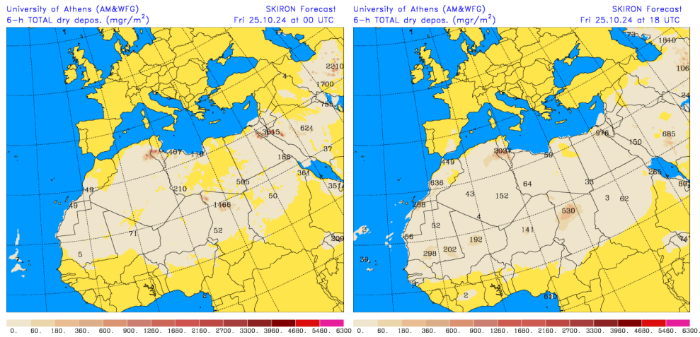
Depósito seco de polvo (mg/m 2 ) predicho por el modelo SKIRON para el día 25 de octubre de 2024 a las 00 y 18 UTC © Universidad de Atenas.
