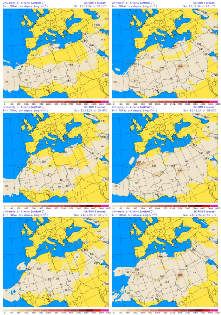
Depósito seco de polvo ( \text{mg}/\text{m}^2 ) predicho por el modelo SKIRON para los días 21, 22 y 23 de diciembre de 2024 a las 00 y 18 UTC © Universidad de Atenas.
