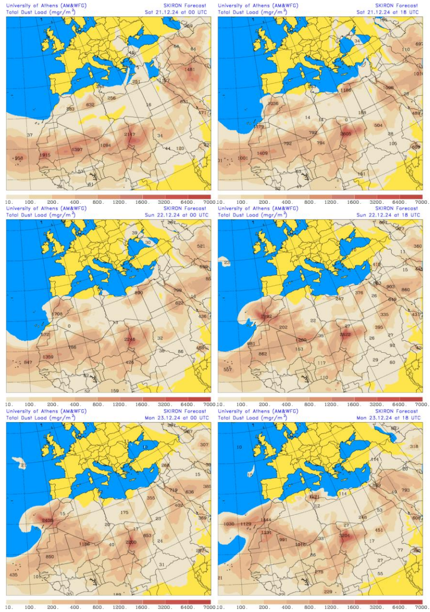
Carga total de polvo ( \text{mg}/\text{m}^2 ) predicha por el modelo SKIRON para los días 21, 22 y 23 de diciembre de 2024 a las 00 y 18 UTC © Universidad de Atenas.
