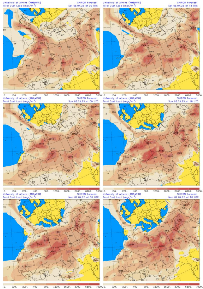
Carga total de polvo (mg/m 2 ) predicha por el modelo SKIRON para los días 5, 6 y 7 de abril de 2025 a las 00 y 18 UTC © Universidad de Atenas.
