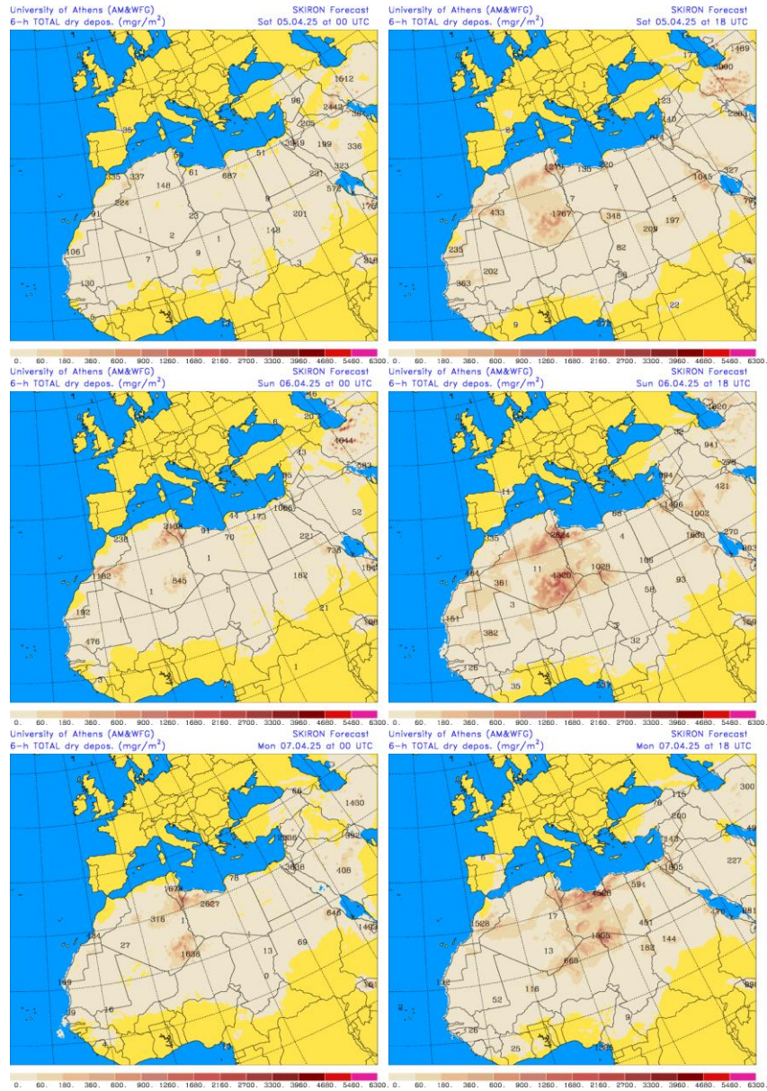
Depósito seco de polvo ( \text{mg}/\text{m}^2 ) predicho por el modelo SKIRON para los días 5, 6 y 7 de abril de 2025 a las 00 y 18 UTC © Universidad de Atenas.
