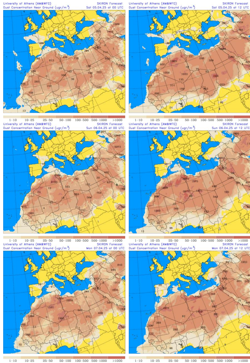
Concentración de polvo ( \mu\text{g}/\text{m}^3 ) predicha por el modelo SKIRON para los días 5, 6 y 7 de abril de 2025 a las 00 y 12 UTC © Universidad de Atenas.
