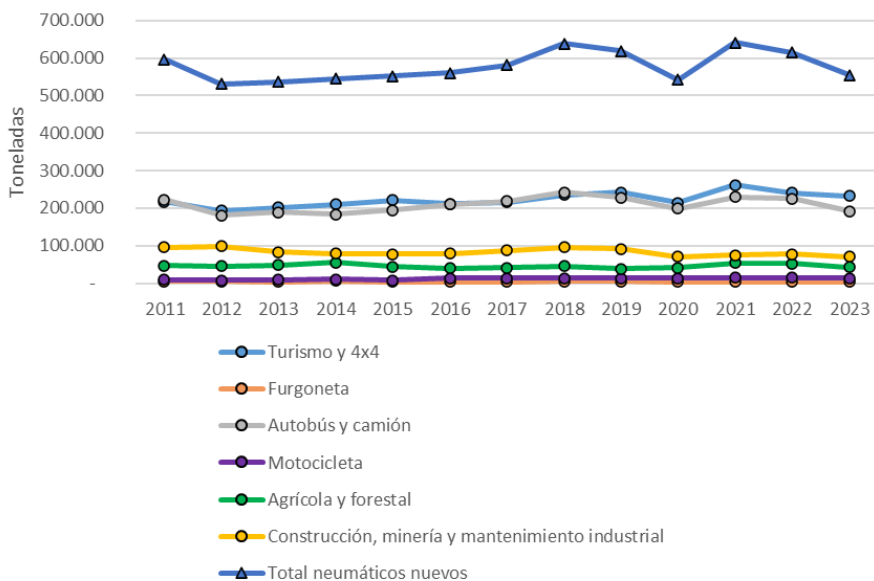
Evolución de la exportación de neumáticos nuevos
