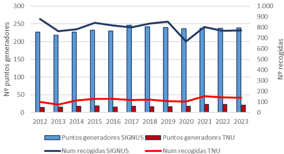
Evolución puntos generadores y número de recogidas en La Rioja
