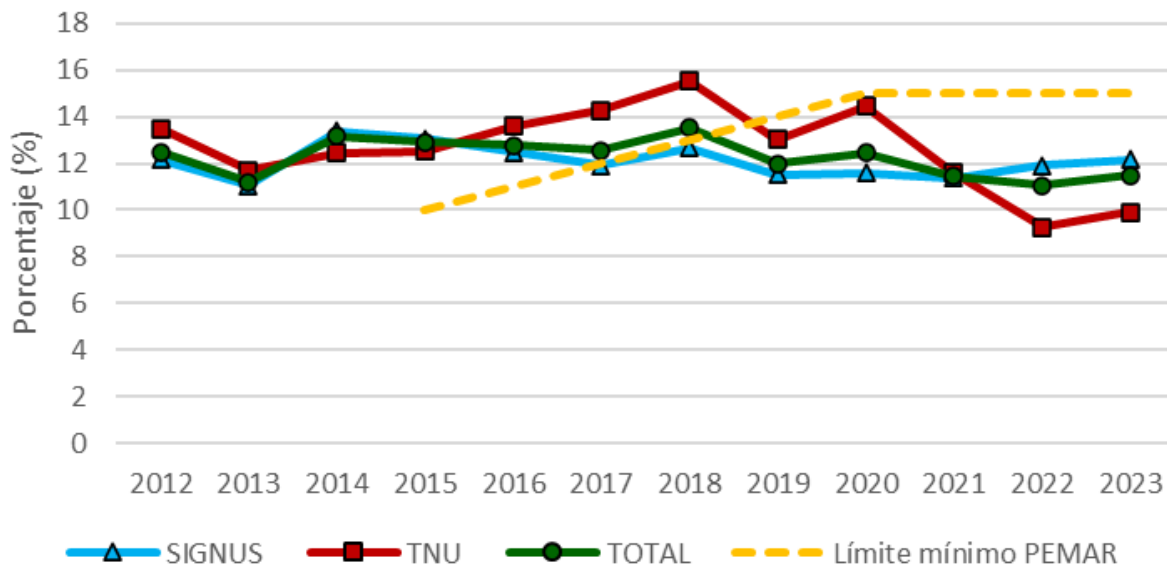
Evolución de la relación entre preparación para la reutilización y recogida NFU
