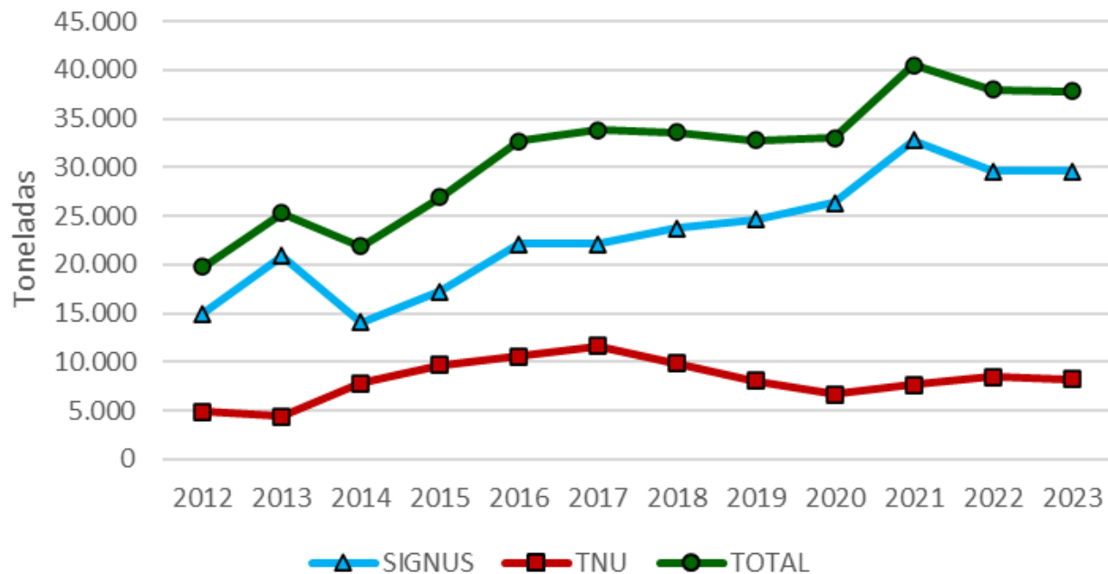
Acero reciclado puesto en el mercado
