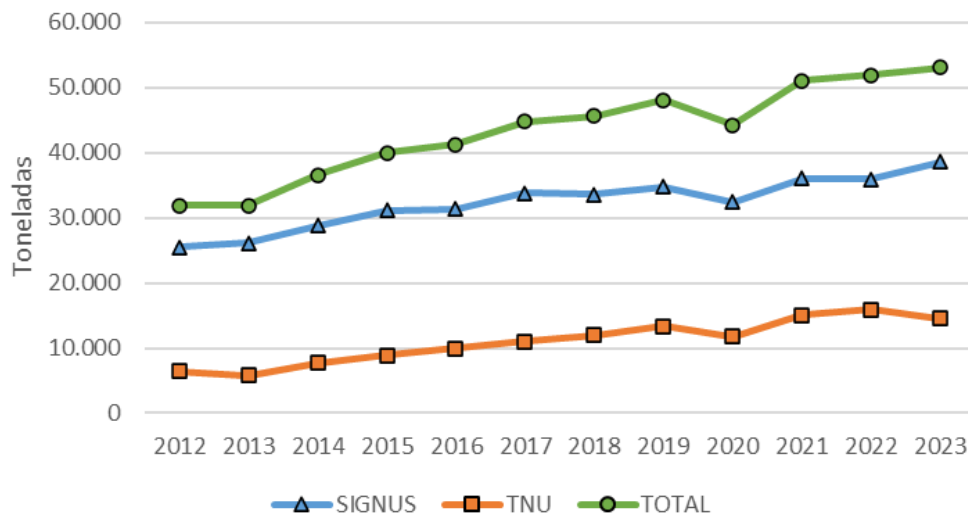
Evolución recogida NFU en Andalucía
