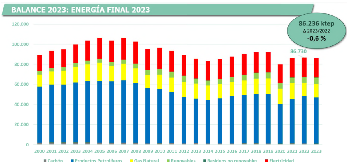
Figura 1.4. Consumo de energía final, incluyendo usos no energéticos, 2000-2023
