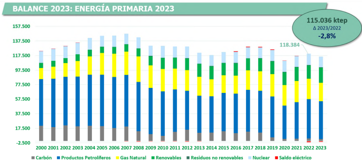
Figura 1.2. Consumo de energía primaria 2000-2023
