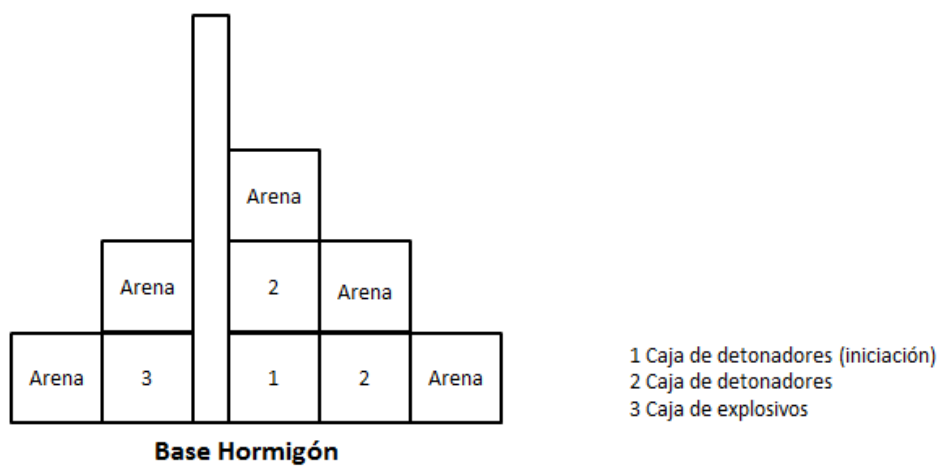
Figura 1: Alzado
