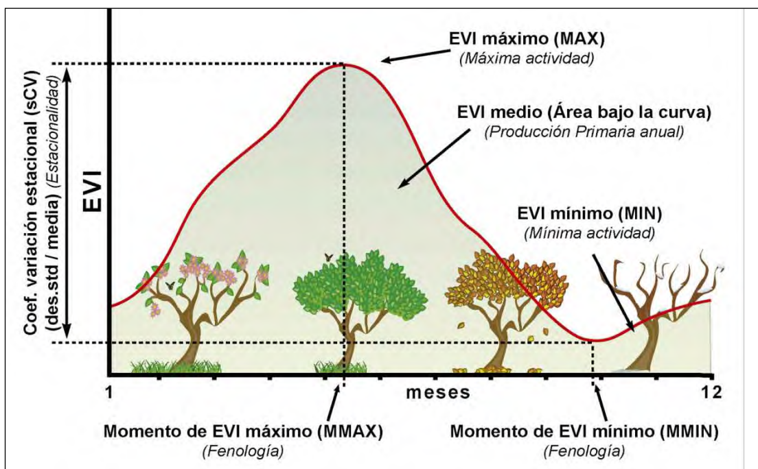
Figura 03. Curva anual índice de verdor. Dinámica del índice de verdor (EVI o NDVI) e indicadores del funcionamiento derivados de su parametrización. Cabello, J., Reyes, A.
